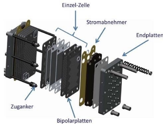
Brennstoffzellen-Stapel
